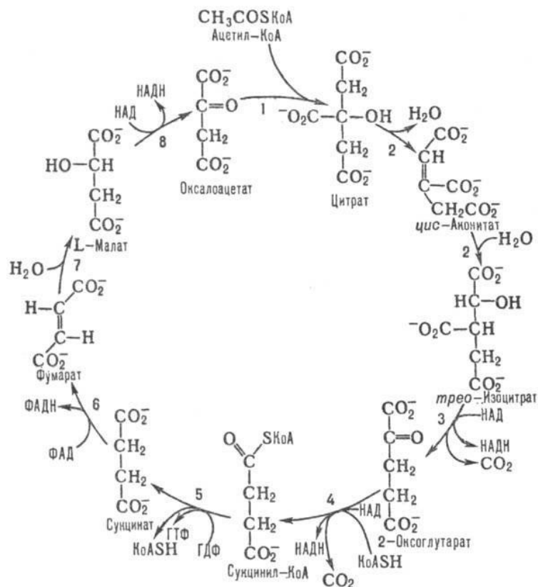
Рис. 1. Крикл Кребса
