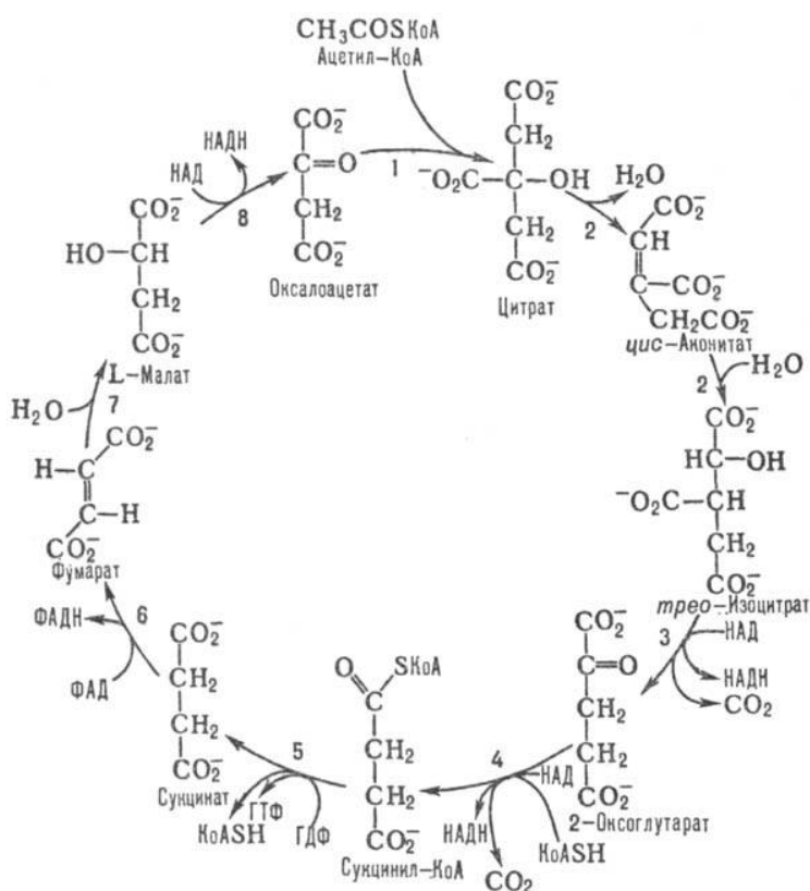
Рис. 1. Цикл Кребса
