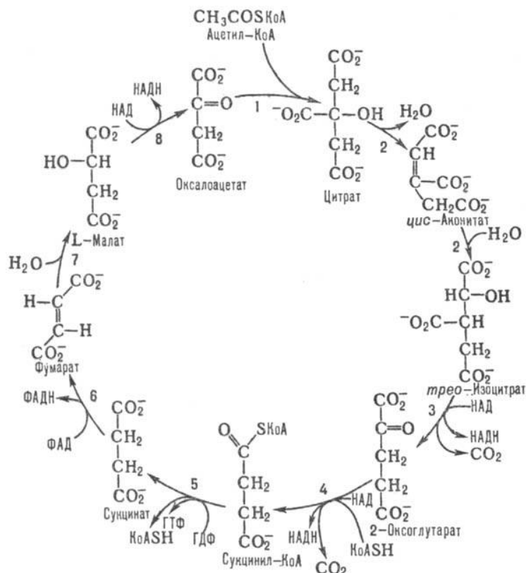
Рис. 1. Цикл Кребса
